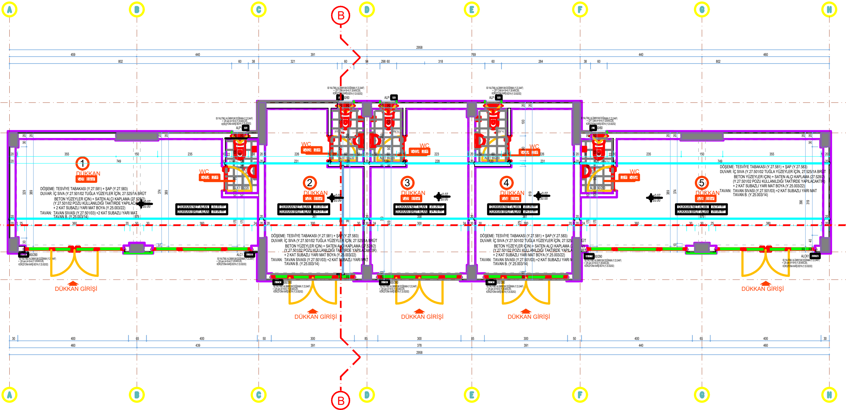
TİCARET BİRİMİ 7 DÜKKAN ZEMİN KAT PLANI Ölçek:1/50
